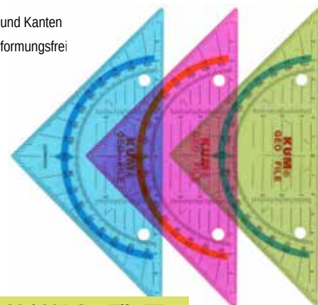
208.19.29 / 261 GeoFile TB
